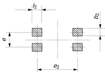
Zones de contact des sorties
