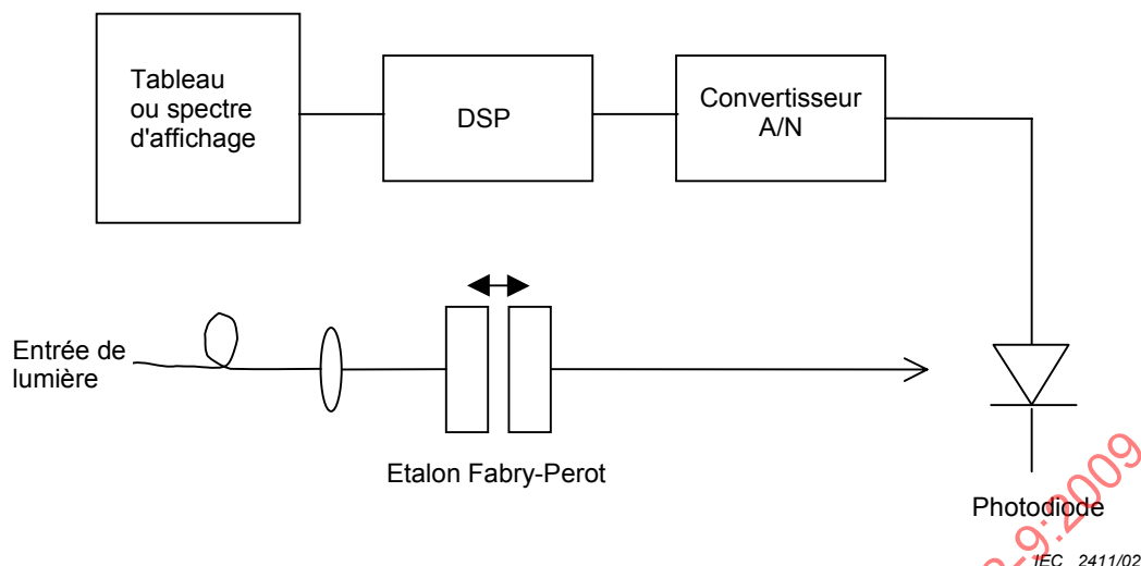
Figure 5 – OSA réalisé à partir d'un Fabry-Perot
