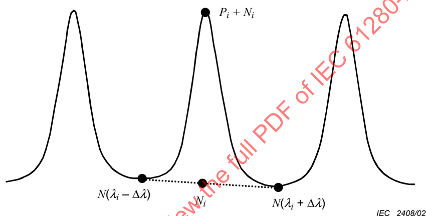
Figure 2 – OSNR de chaque voie, dérivé des mesures directes du spectre optique
