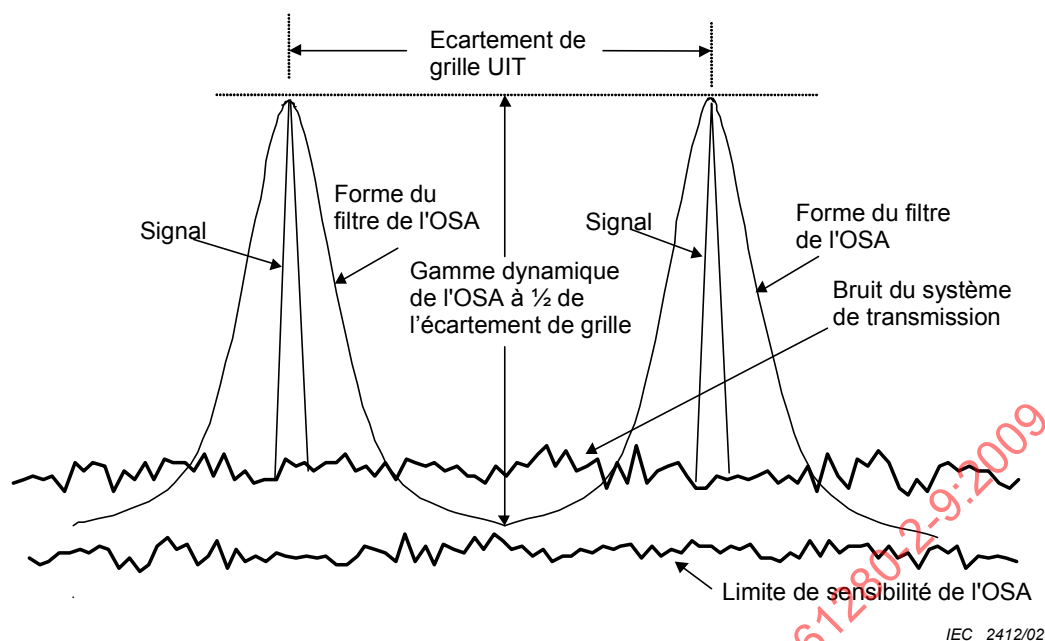
Figure 6 – Illustration de l'insuffisance de la plage dynamique comme autre source d'incertitude de mesure
